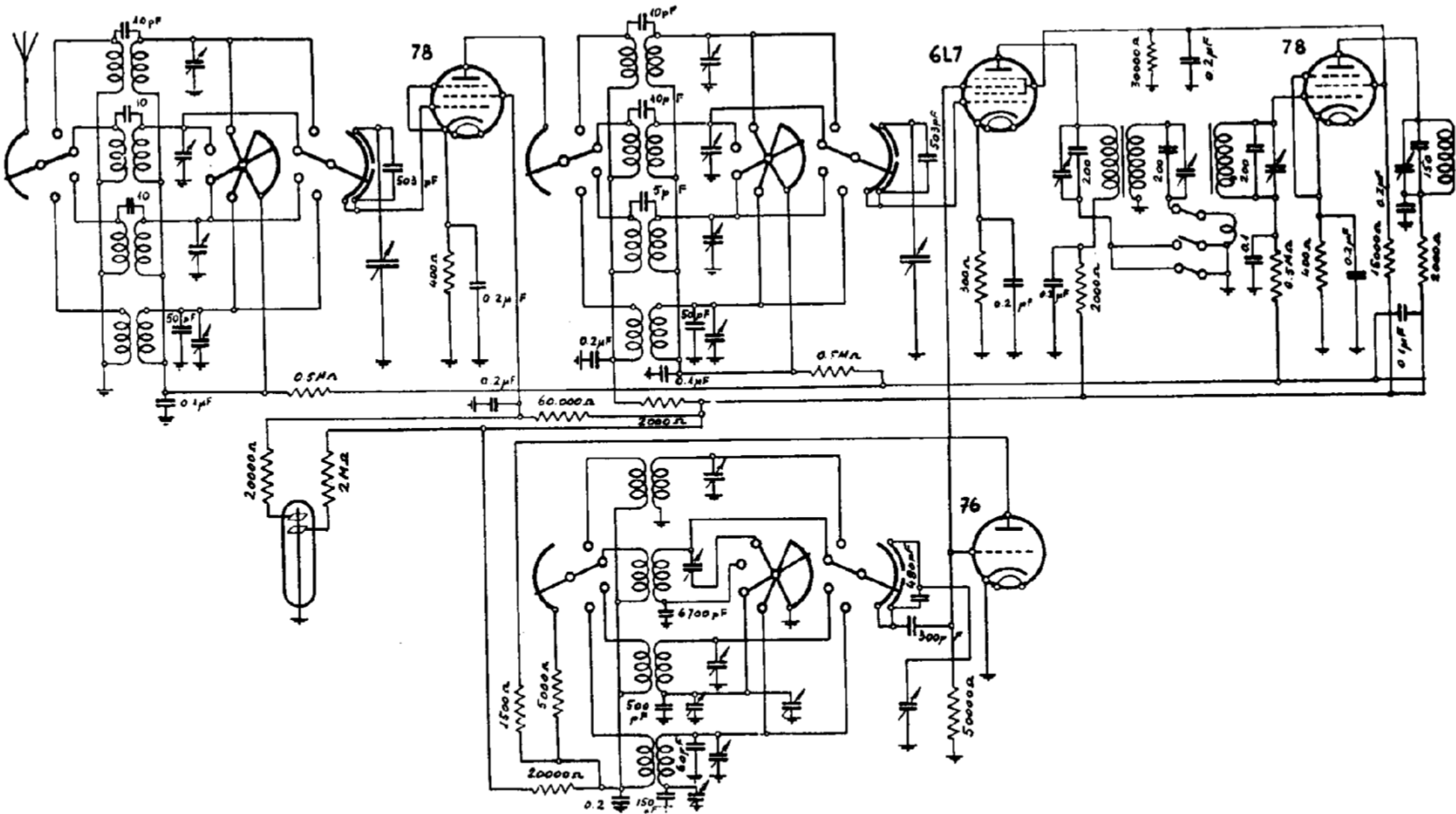
RADIO SAFAR. — Mod. « 844 » e « 940 ». — Parte amplificatrice ad alta e media frequenza (V. nelle pagine seguenti le altre parti). Media frequenza: \text{ZH}\text{X} 094 — Gamme: c. c. (95-19 MHz), c. (55-10 MHz), m. (520-1500 kHz), l. (140-300 kHz).
